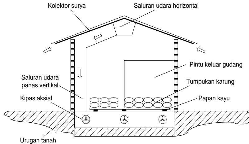
Gbr. 5. Gudang Penyimpanan Dengan Atmosfir Terkendali (Sumber : Mulato, S.dkk, 2003)
