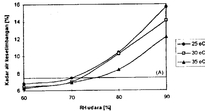
Gbr. 3. Kadar air kesetimbangan biji kakao kering pada berbagai kondisi udara
