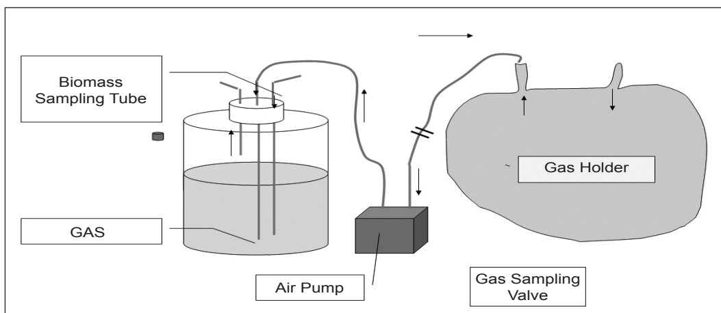
Gambar 1. Skema Fotobioreaktor
