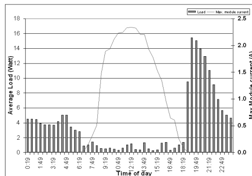
Gambar 2. Arus modul maksimum dan arus beban rata-rata di bulan November
