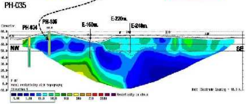
Gambar 8 : Penampang Model Resistivity Pada Lintasan P-07 Dan Data Bor PH-035.
