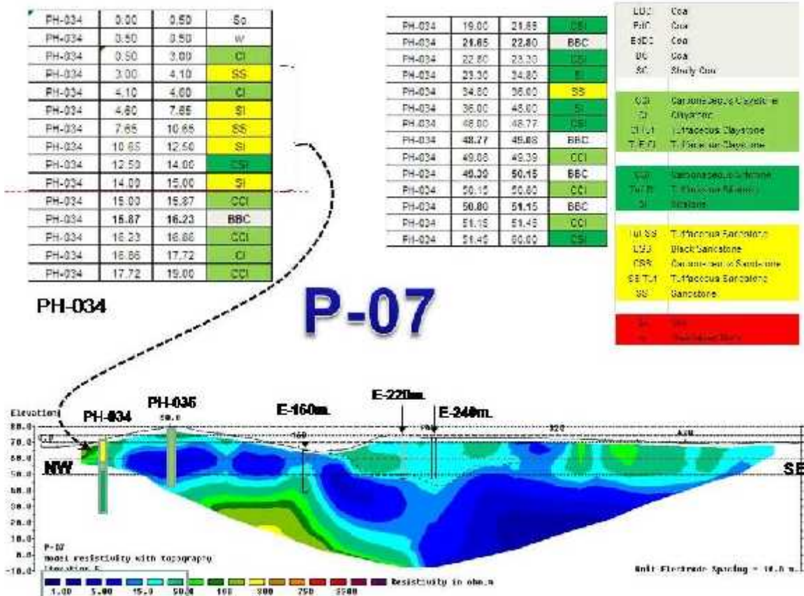
Gambar 7 : Penampang Model Resistivity Pada Lintasan P-07 Dan Data Bor.
