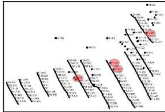
Gambar 5 :Sebaran Data Bor Dan Lintasan Pengukuran Geolistrik2D.
