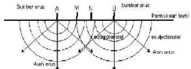
Gambar 2 : Arah Arus Listrik Dan Garis Equipotensial Untuk Dua Sumber Arus Berada Di Permukaan Bumi.
