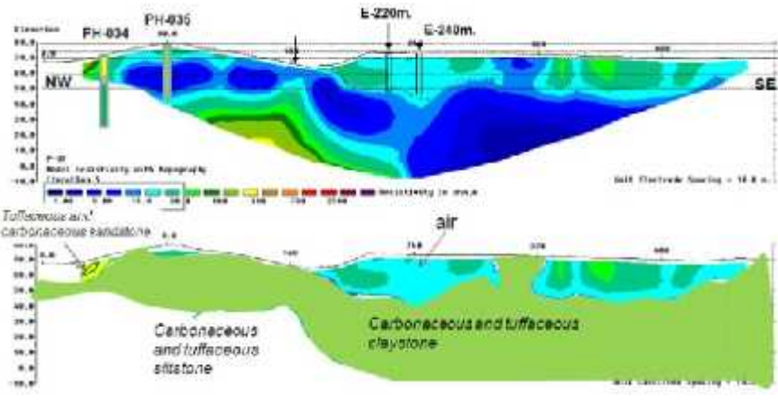
Gambar 9 : Penampang Model Resistivity Pada Lintasan P-07 Dan Interpretasi Geologi.
